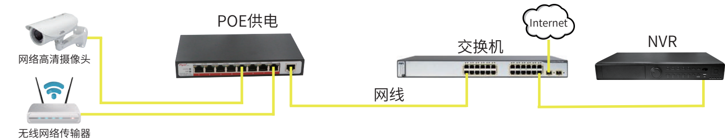
产品连接图
